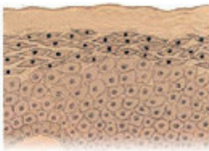
人类皮脂结构
